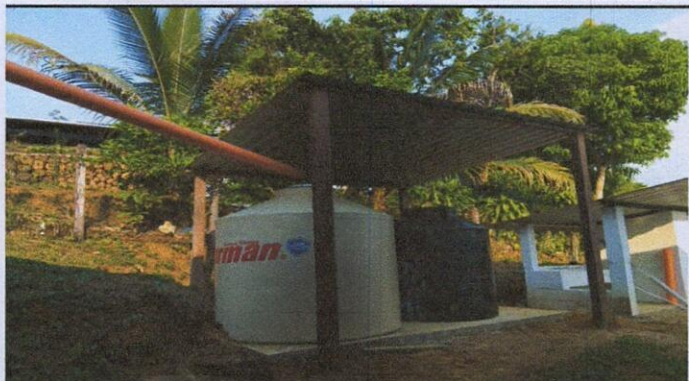
Foto1: Canales y bajada de agua Pluvial
